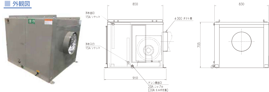
■ 外観図
