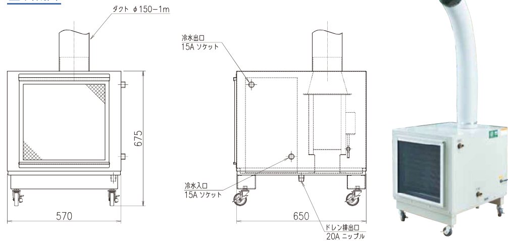
■ 外観図
