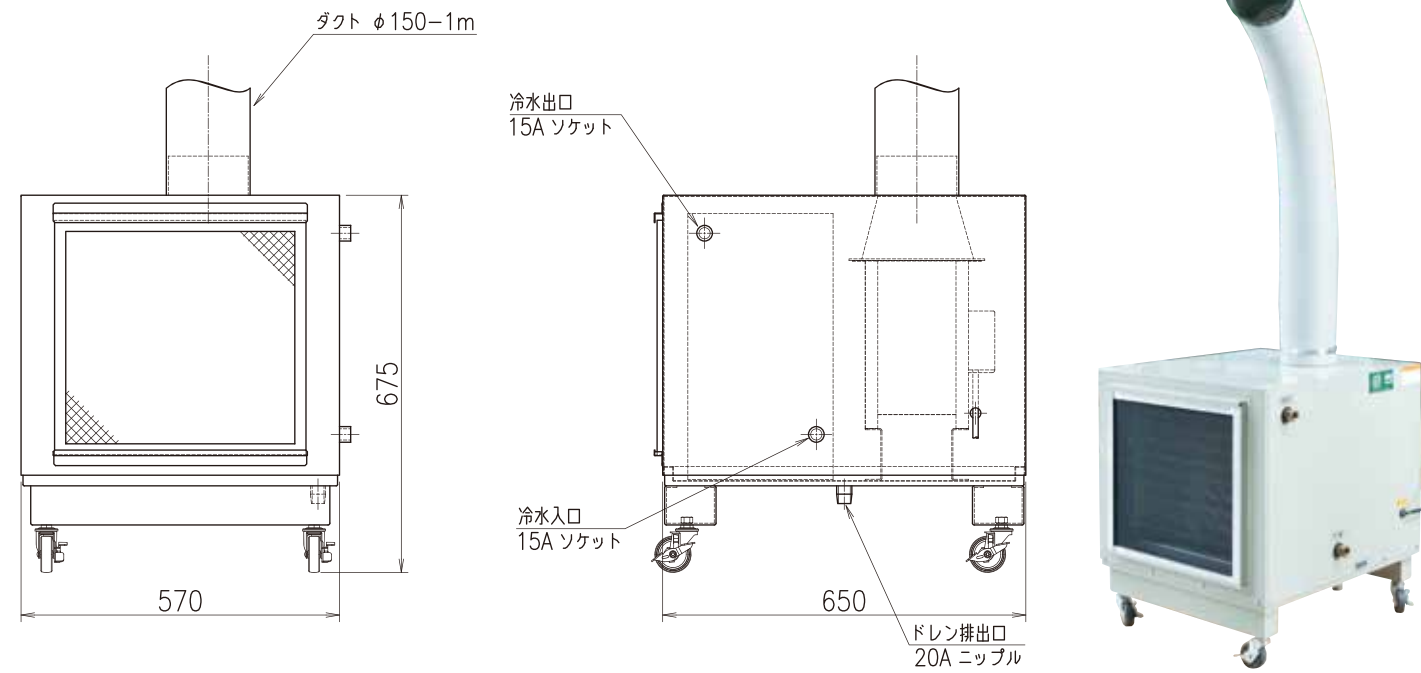
■ 外観図
